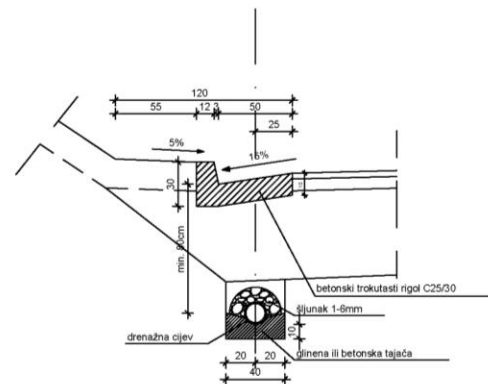
DETALJ DRENAŽE MJ 1:25
